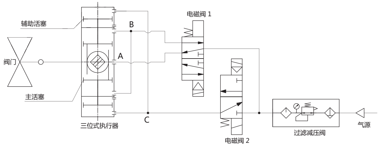
三位式气动执行器工作原理图
