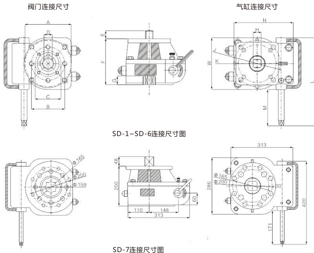
SD系列气动阀门手操机构连接尺寸表
